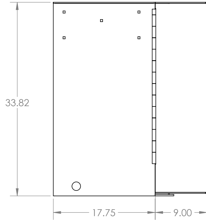
LEFT SIDE
